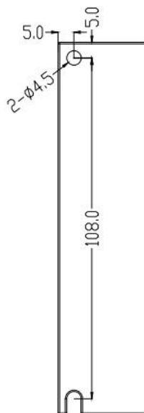
图 2-1 CL3J-EC503/CL3J-EC507 安装尺寸图(单位: mm)
