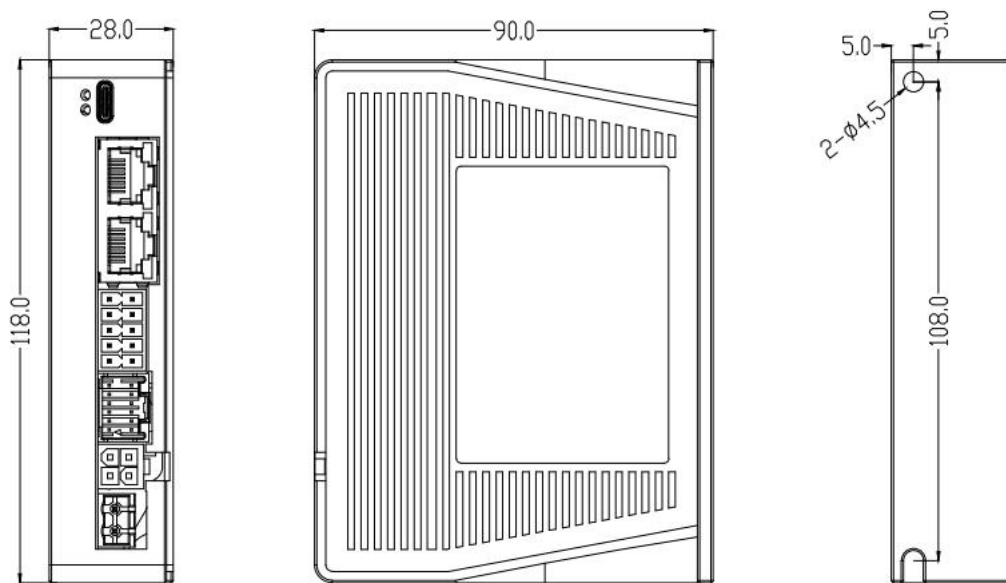
图 2-1 CL3J-EC503/507 安装尺寸图(单位: mm)
